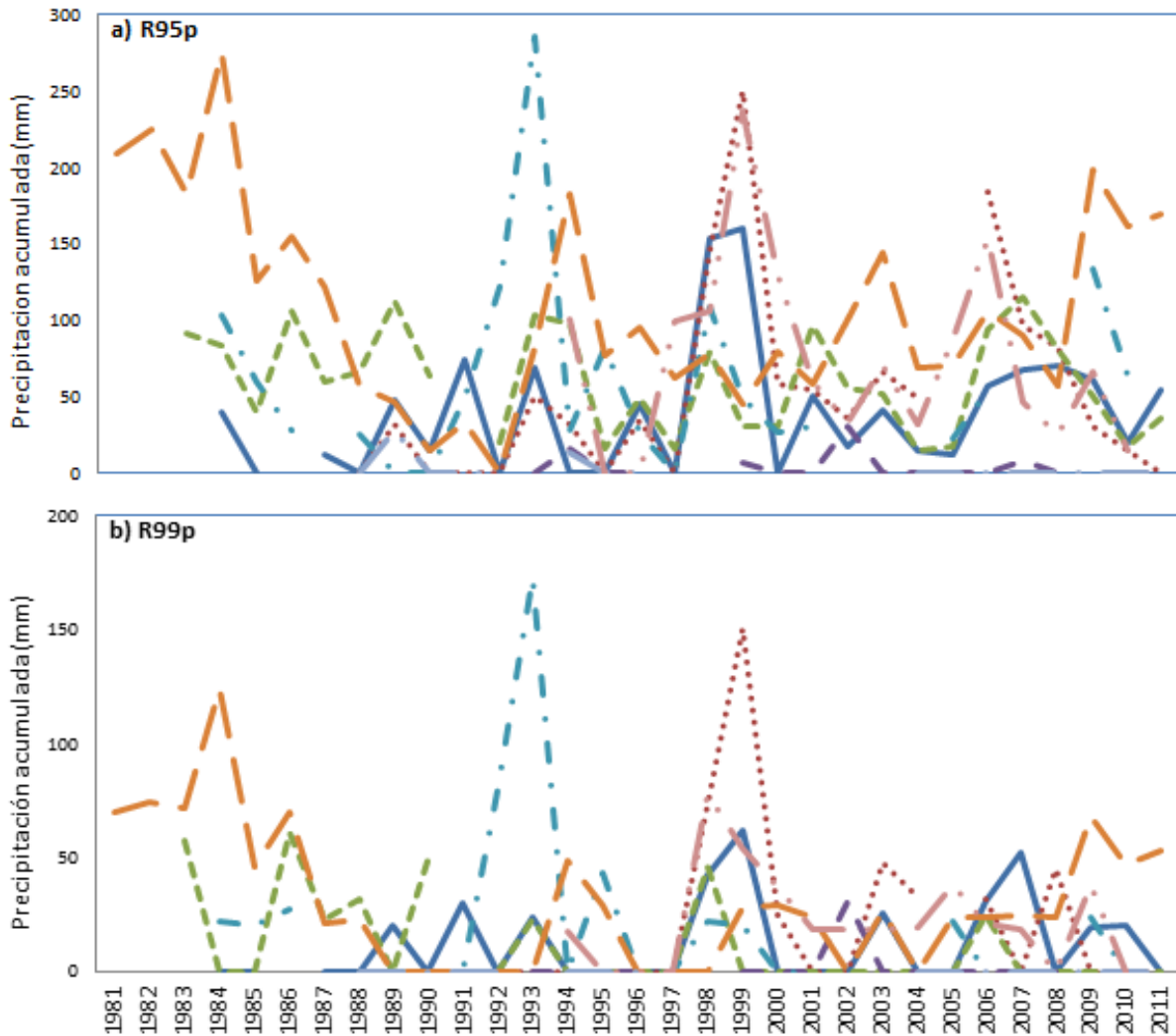
Figura 3. (a) Precipitación acumulada (mm) de los días que se supera el percentil 95 del periodo 1981-2012. (b) Precipitación acumulada (mm) de los días que se supera el percentil 99 del periodo 1981-2012. Cada línea indica una estación; Autisha (línea sólida), Canchacalla (línea punto-redondo), Carampoma (línea punto-cuadrado), Chosica (línea guion), Matucana (línea guion-punto), San José de Parac (línea guion largo), Santa Eulalia (línea guion largo-punto), Sheque (línea guion-punto-punto). Elaborado: Dirección Regional de Lima.
